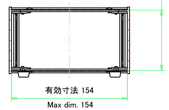
C-C ( 1 : 3 )
