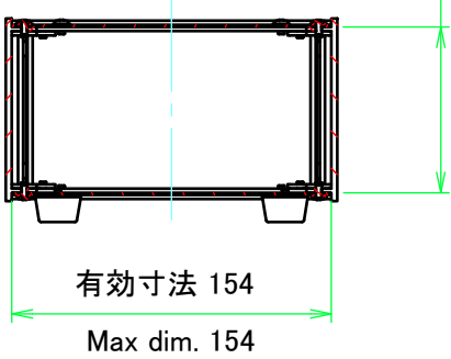
C-C ( 1 : 4 )
