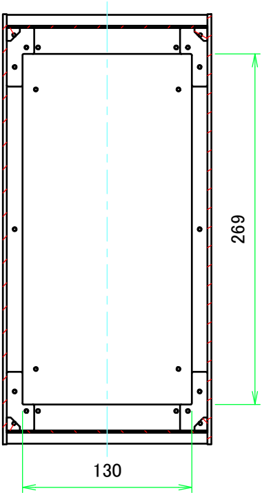
B-B ( 1 : 4 )
