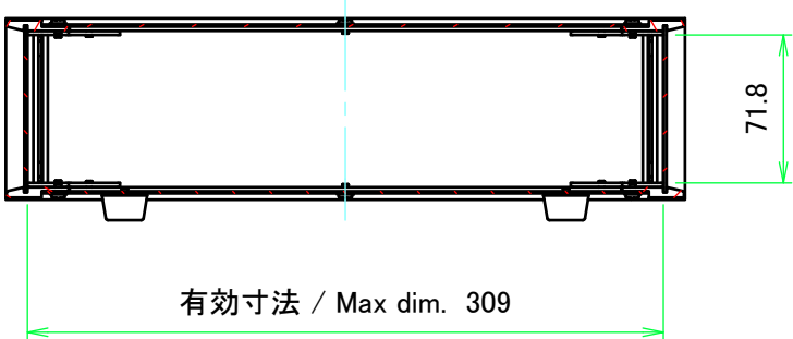
A-A ( 1 : 4 )
