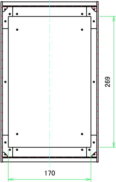
B-B ( 1 : 4 )
