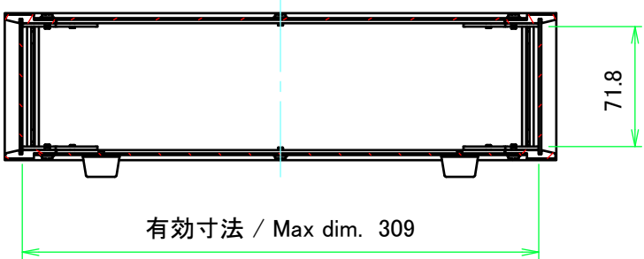
A-A ( 1 : 4 )
