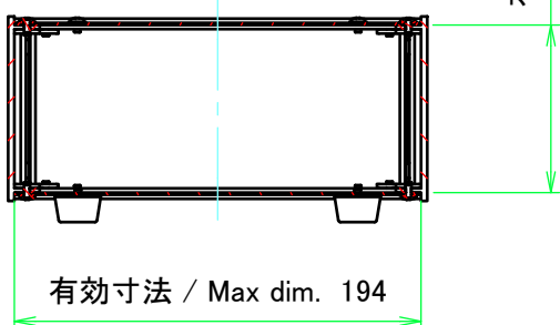
C-C ( 1 : 4 )
