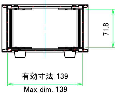
A-A ( 1 : 4 )
