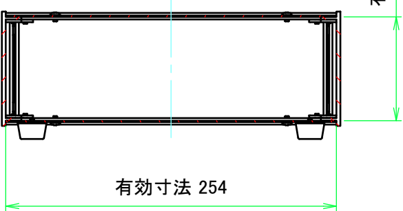
C-C ( 1 : 4 )
