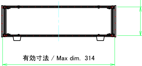
C-C ( 1 : 5 )
