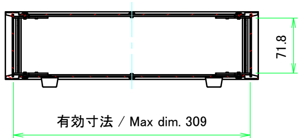
A-A ( 1 : 5 )
