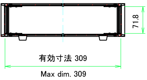
A-A ( 1 : 6 )
