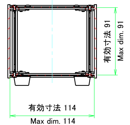
C-C ( 1 : 3 )
