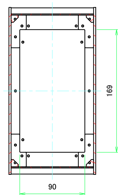
B-B ( 1 : 3 )
