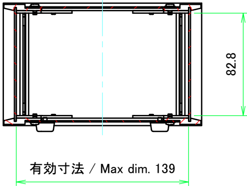
A-A (1:3)
