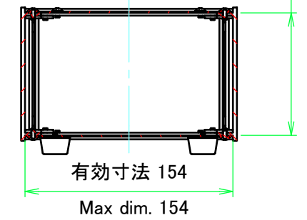
C-C ( 1 : 4 )
