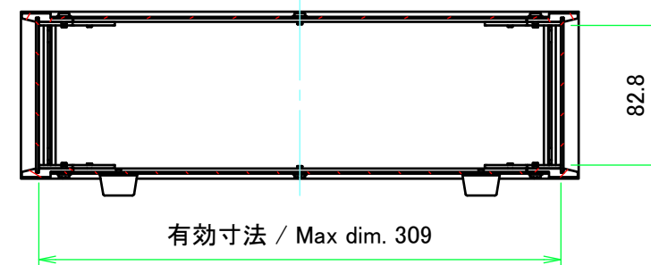
A-A ( 1 : 4 )
