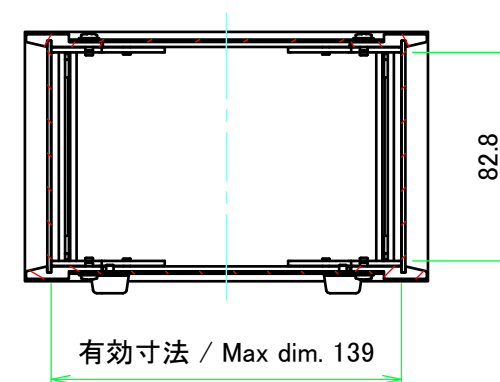
A-A (1:3)
