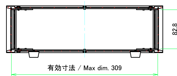
A-A ( 1 : 4 )
