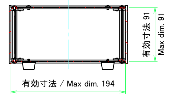
C-C ( 1 : 4 )
