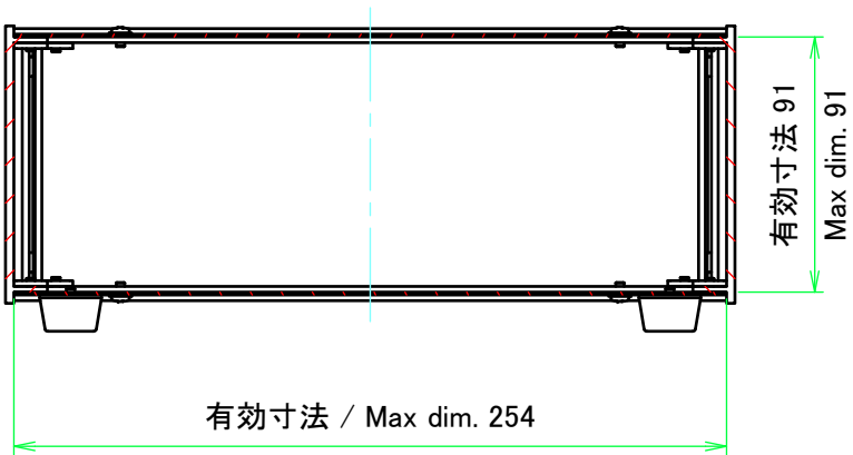
C-C ( 1 : 3 )
