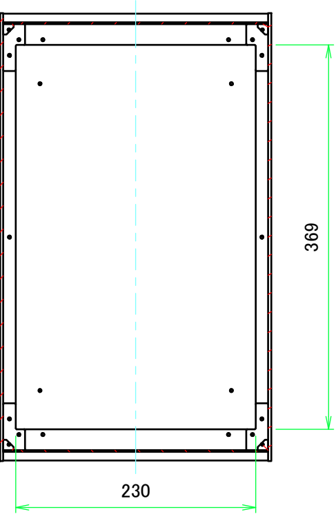
B-B ( 1 : 5 )
