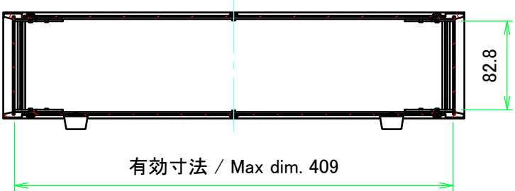
A-A ( 1 : 5 )
