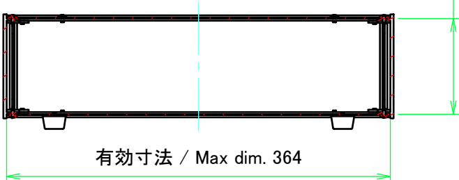
C-C ( 1 : 5 )
