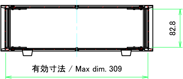
A-A ( 1 : 5 )
