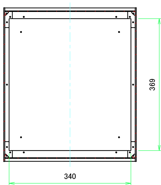
B-B ( 1 : 6 )
