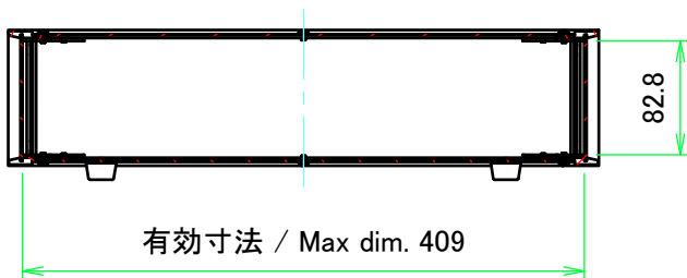
A-A ( 1 : 6 )
