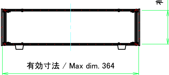
C-C ( 1 : 6 )
