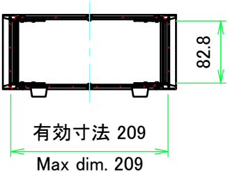
A-A ( 1 : 7 )
