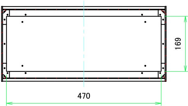
B-B ( 1 : 7 )
