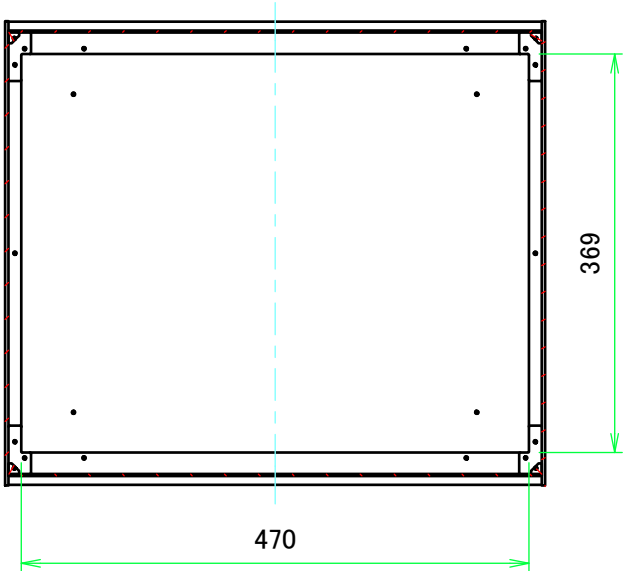
B-B ( 1 : 7 )
