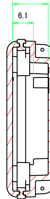
B-B ( 1.5 : 1 ) 有効寸法 / Max dim. 10.4
