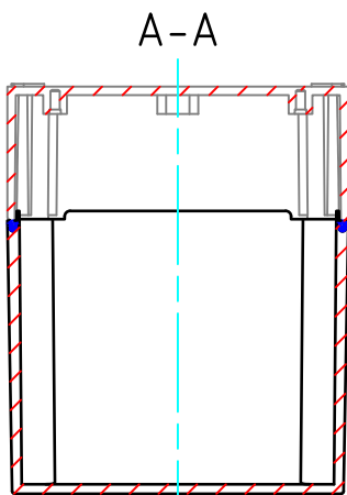
ボディー(内視) BASE (Internal View)
