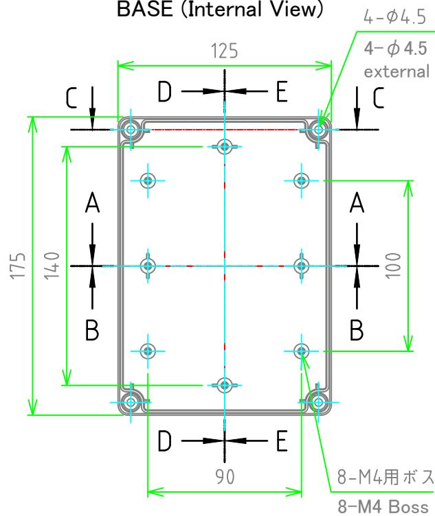
ボディー(内視) BASE (Internal View)
