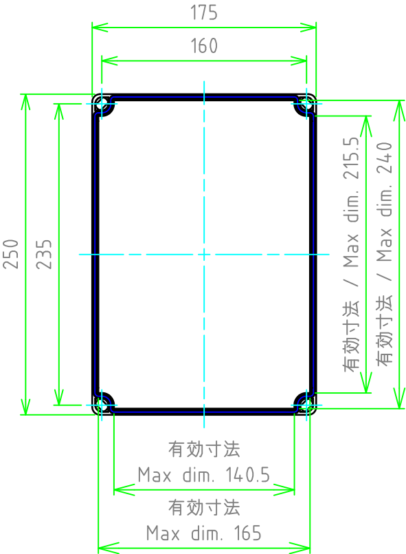
カバー(内視) Cover (Internal View)
