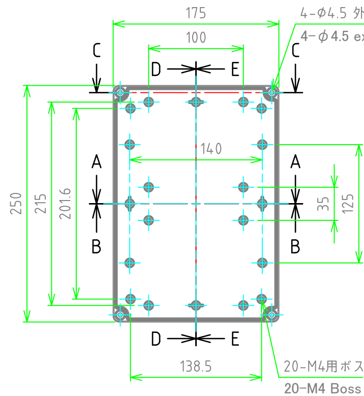
ボディー(内視) BASE (Internal View)
