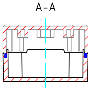
ボディー(内視) Base (Internal View)
