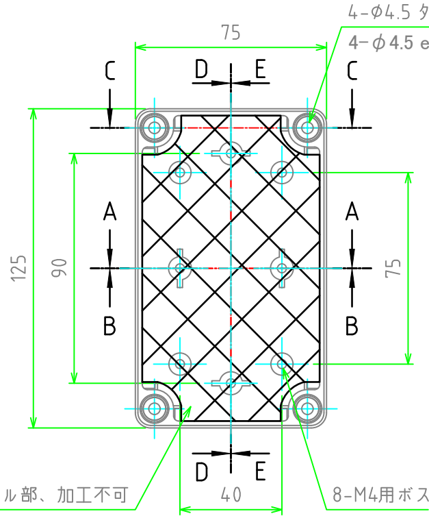
ボディー(内視) Base (Internal View)
