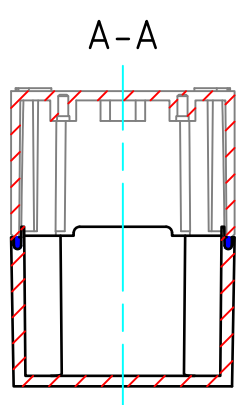
ボディー(内視) Base (Internal View)
