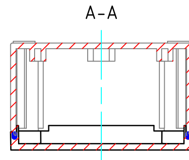
ボディー(内視) BASE (Internal View)
