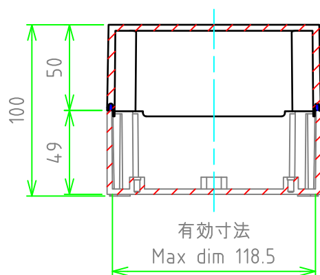
B-B
