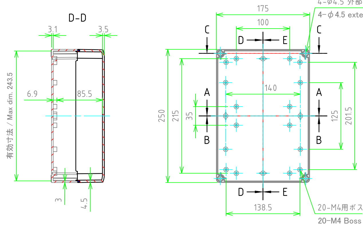
ボディー(内視) BASE (Internal View)
