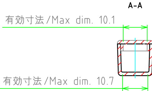
カバー (内視) Cover (Internal View)
