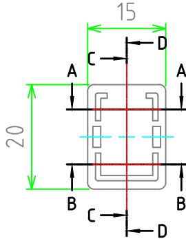
カバー (内視) Cover (Internal View)
