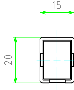
ボディー (内視) Base (Internal View)
