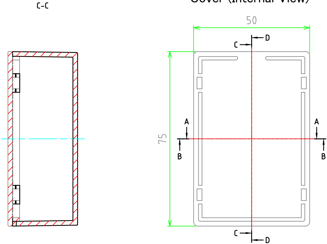
カバー (内視) Cover (Internal View)
