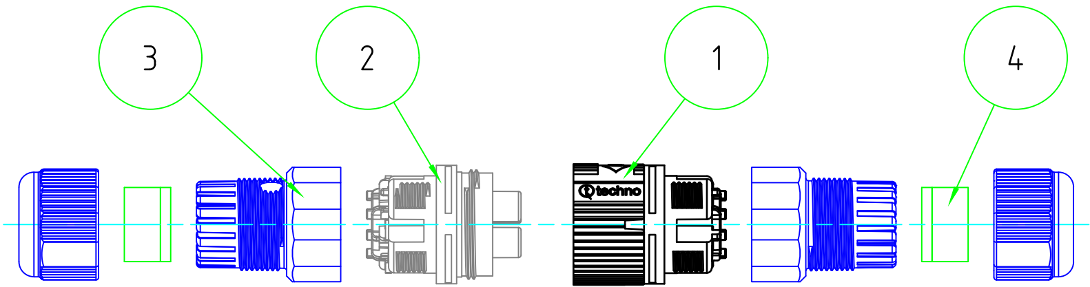
展開図
