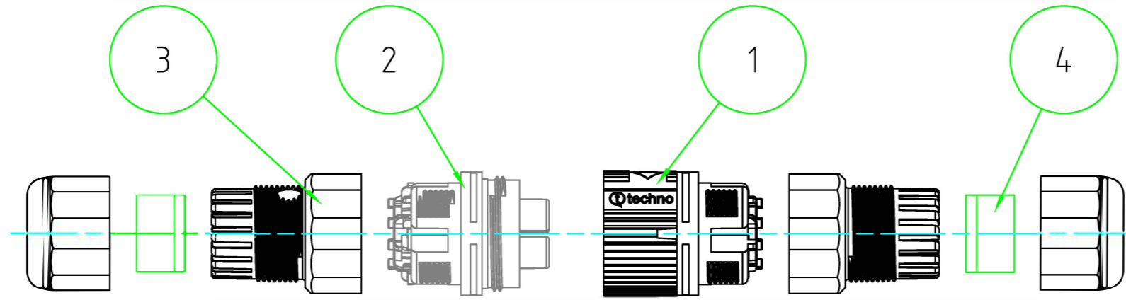
展開図
