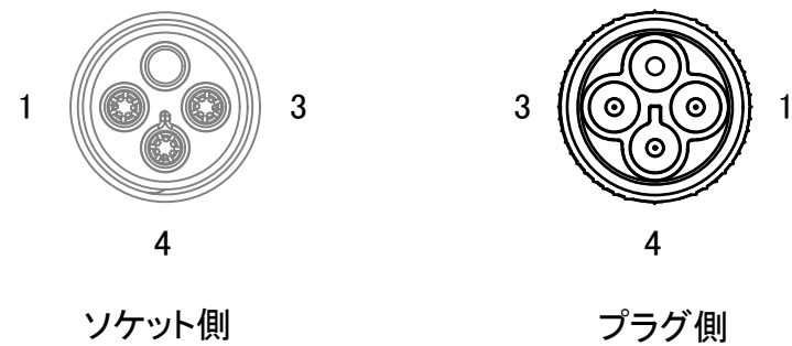
端子配列図
