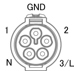
プラグ側
