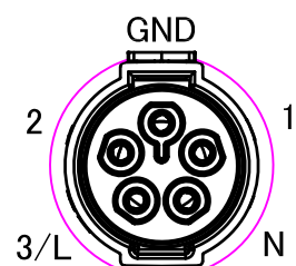
ソケット側
