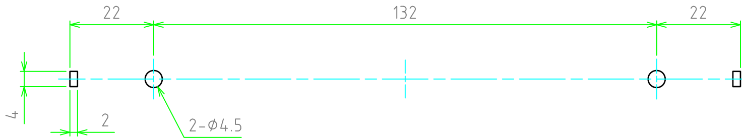
取付穴寸法図
