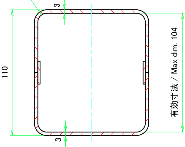
D-D ( 1 : 2 )
