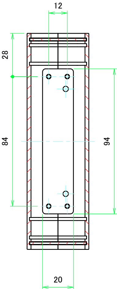
A-A ( 1 : 1.5 )
