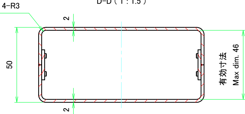
D-D ( 1 : 1.5 )
