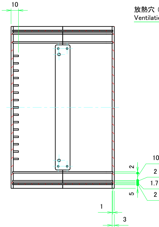
B-B ( 1 : 2.5 )
