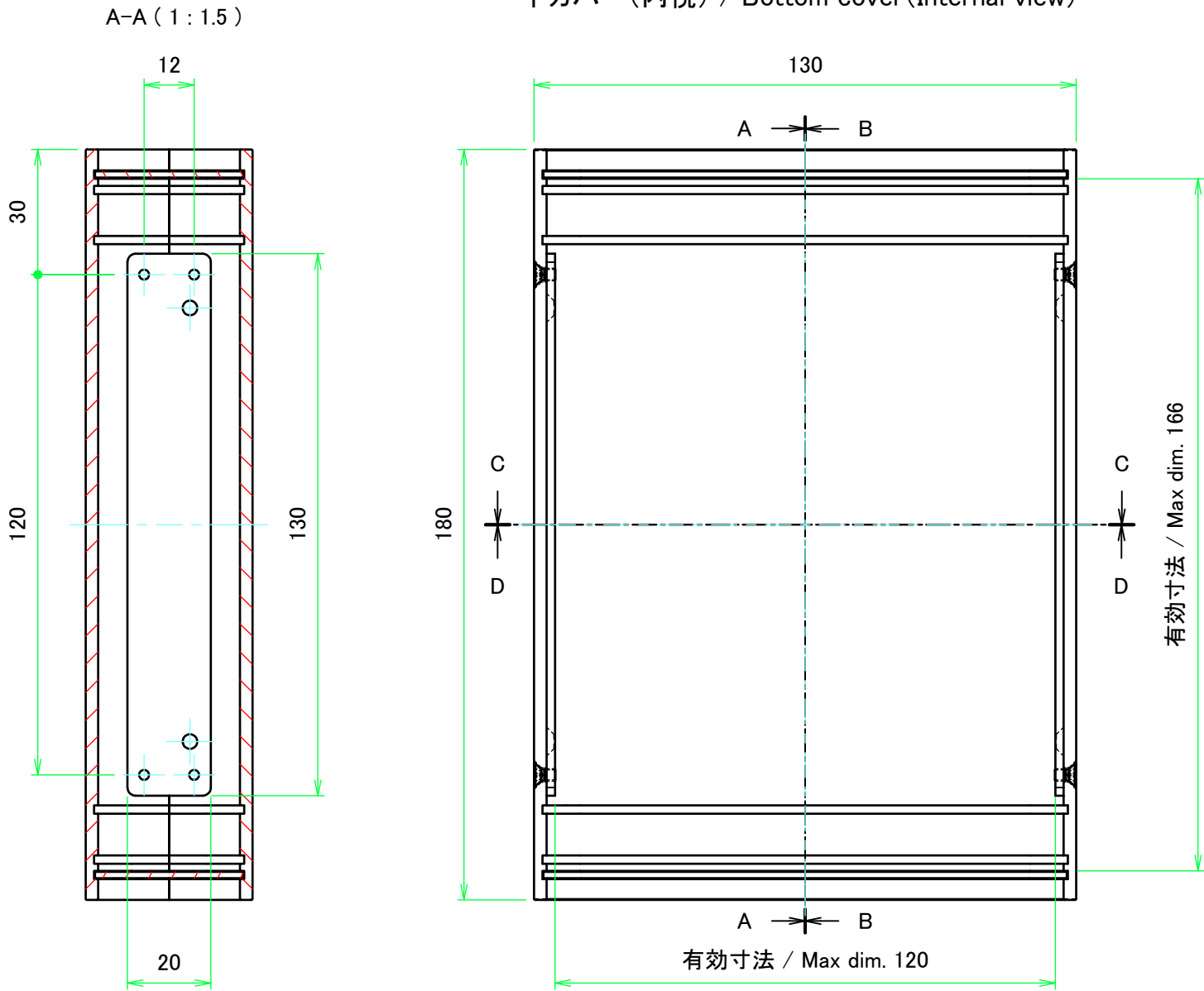
下カバー(内視) / Bottom cover (Internal view)
