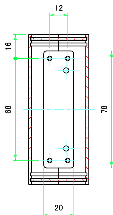
A-A ( 1 : 1.5 )
