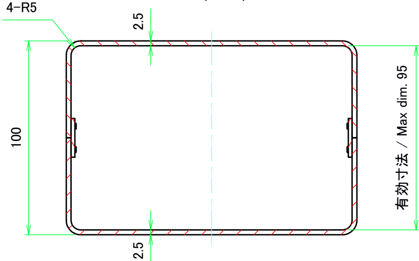
D-D ( 1 : 2 )
