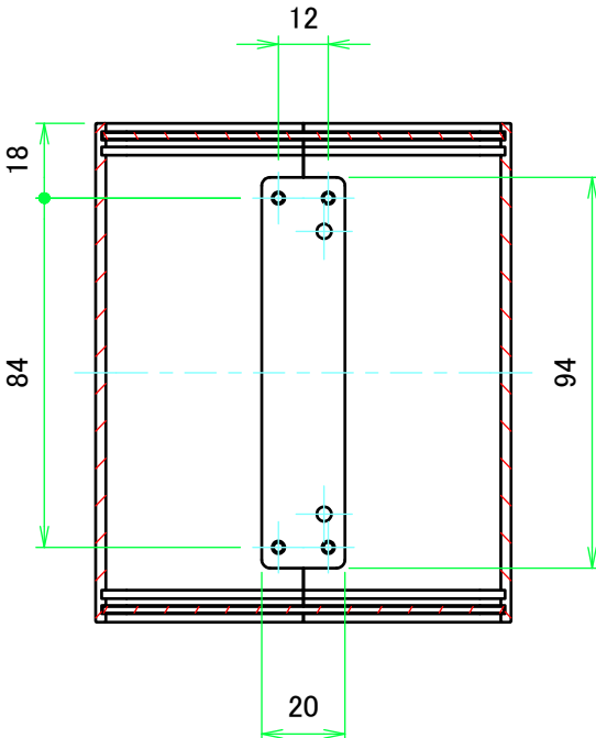
A-A ( 1 : 2
