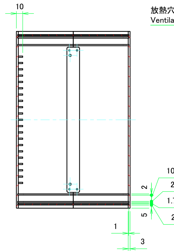
B-B (1:3.5)
