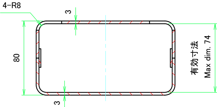
D-D ( 1 : 2.5 )
