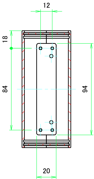
A-A ( 1 : 2 )
