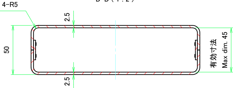
D-D ( 1 : 2 )
