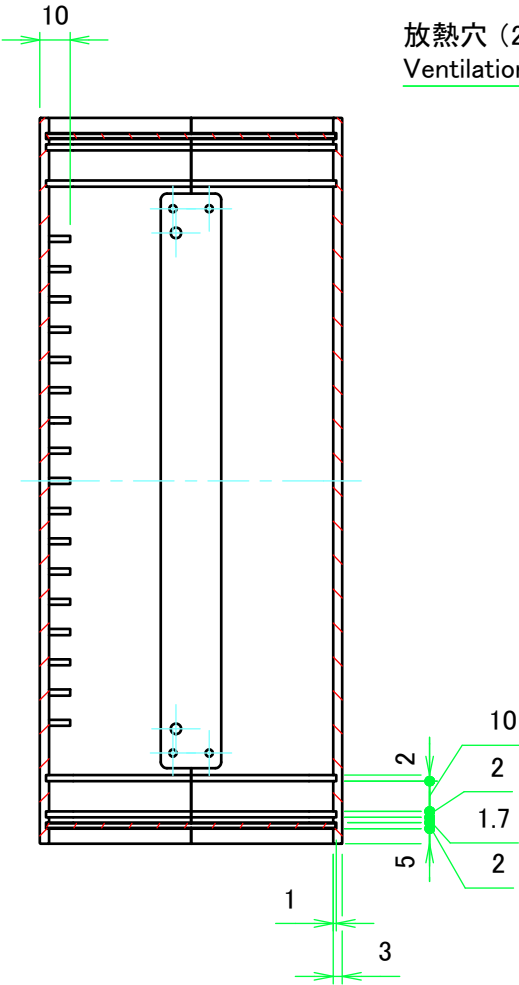
B-B ( 1 : 2.5 )
