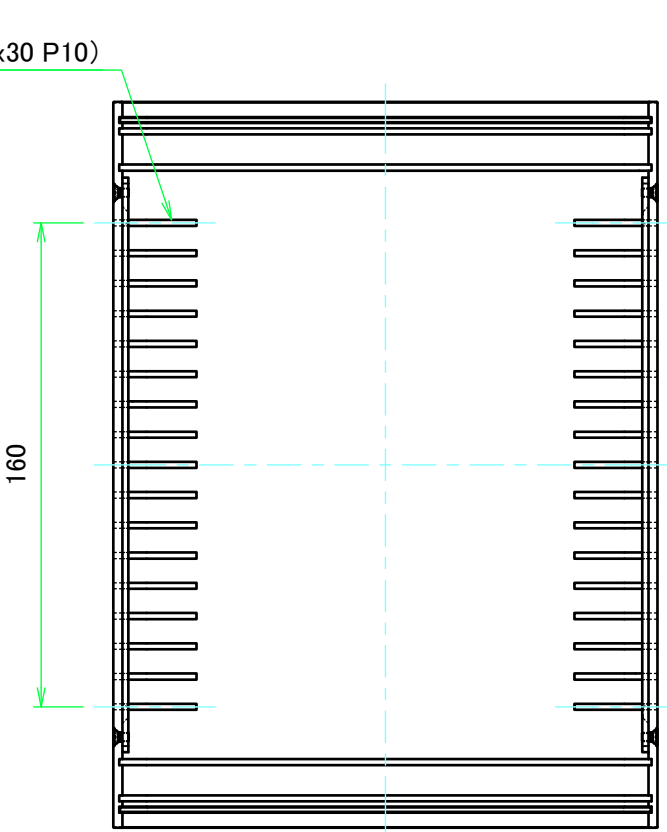
上カバー(内視) Top cover (Internal view)
