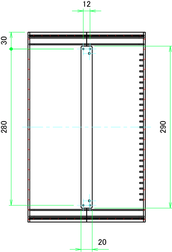
A-A ( 1 : 4 )
