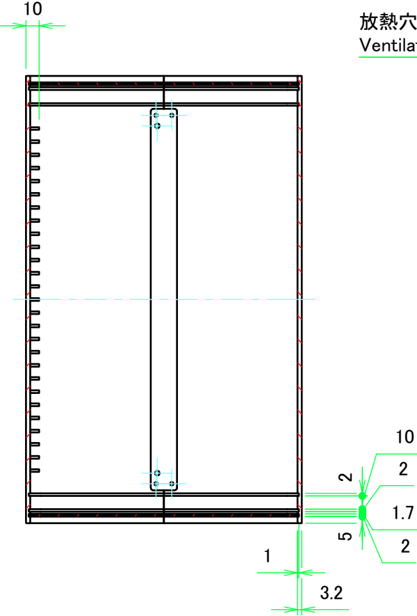
B-B ( 1 : 4 )
