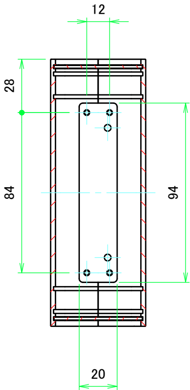
A-A ( 1 : 2 )
