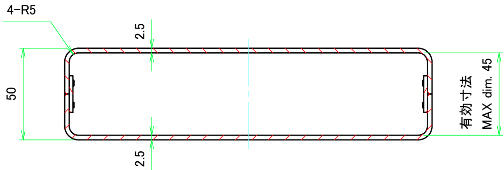
D-D ( 1 : 2 )
