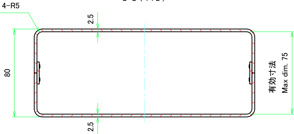
D-D ( 1 : 2 )
