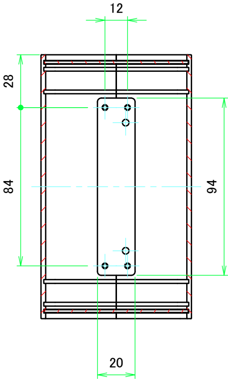
A-A ( 1 : 2 )
