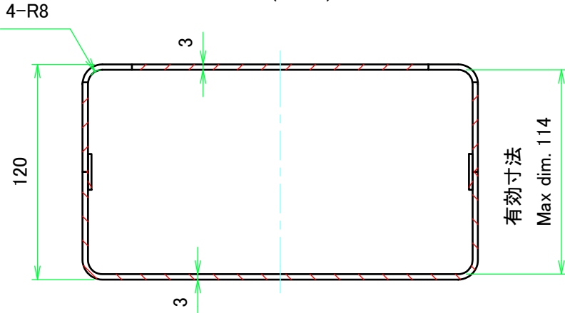
D-D ( 1 : 3 )
