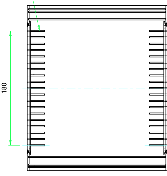
放熱穴 (2x30 P10) Ventilation slits (2x30 P10)
