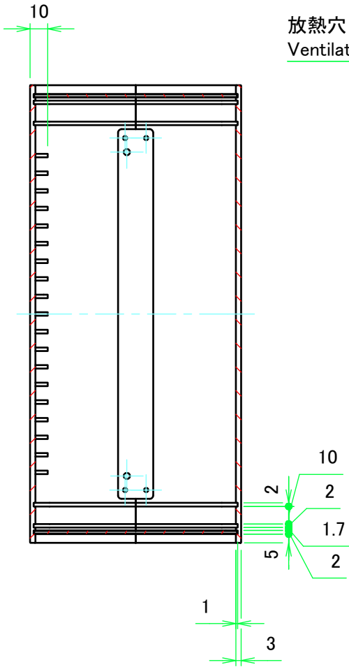
B-B ( 1 : 3 )
