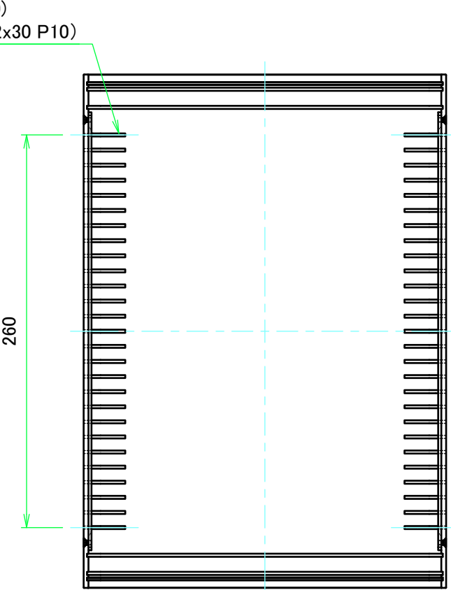
上カバー(内視) Top cover (Internal view)
