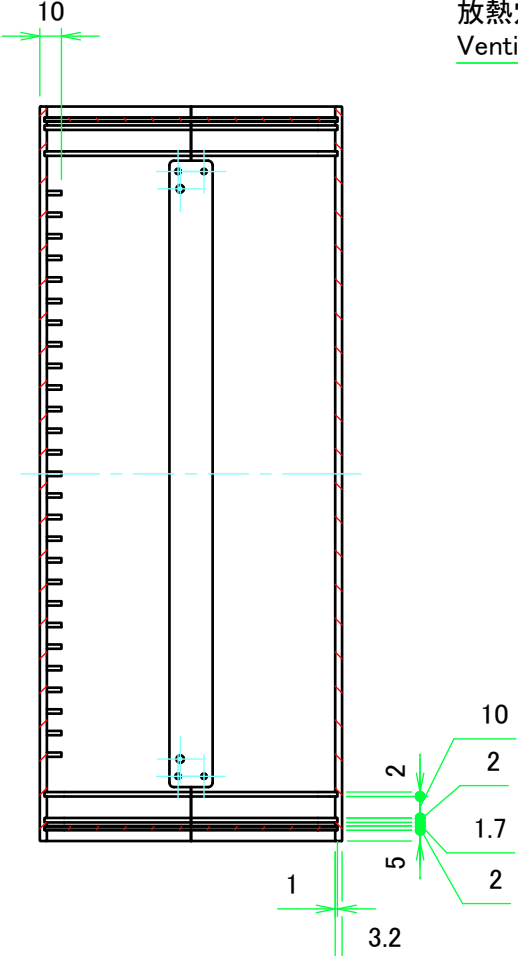
B-B ( 1 : 3.5 )
